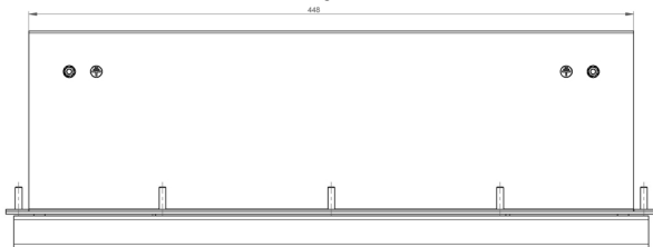
Schublidentastatur im ausgezogenen Zustand
