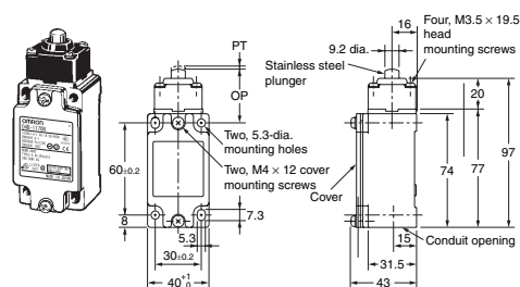
Top Plunger D4B-□□70N
