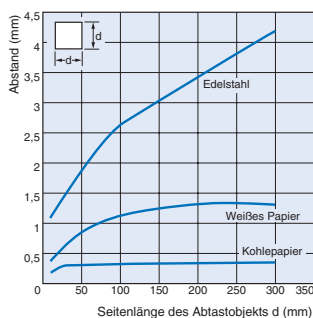
Energetische Reflexionslichttaster E3Z-D□2(D□7)
