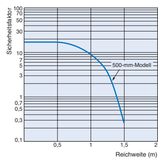
Reflexionslichtschranken für lichtdurchlässige Objekte E3Z-B□1/B□6 + E39-R1S (optionaler Reflektor)
