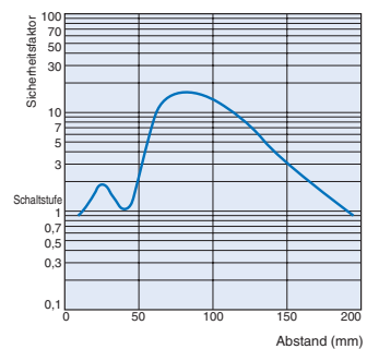
Enger Strahlkegel E3Z-L
