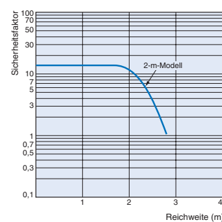
E3Z-B□2/B□7 + E39-R1S (optionaler Reflektor)
