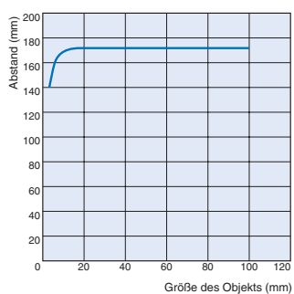
Enger Strahlkegel E3Z-L
