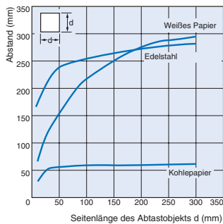
Energetische Reflexionslichttaster E3Z-D□1(D□6)
