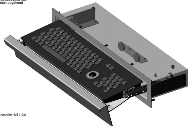
Ohne Anschlußkabel gezeichnet. Kabelausgang nach unten abgehend
