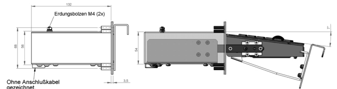
Ohne Anschlußkabel gezeichnet. Kabelausgang nach unten abgehend
