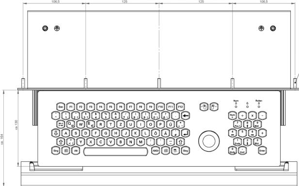
Schubladentastatur im ausgezogenen Zustand
