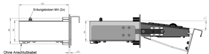
Ohne Anschlußkabel gezeichnet. Kabelausgang nach unten abgehend
