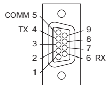
RS-232 DB9-M
