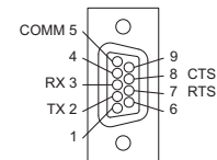
RS-232 DB9-M
