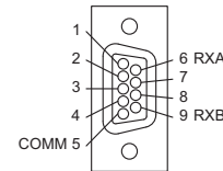
RS-485 DB9-F
