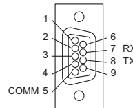
RS-232 DB9-F
