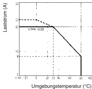
G3PA-420B-VD, G3PA-420B-VD-2
