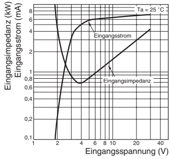
G3PA-2□0B-VD
