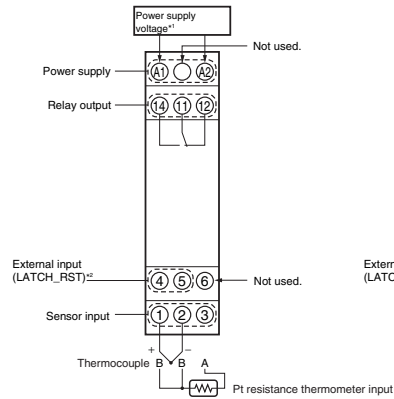
K8AK-TH11S
