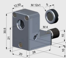
Freiblasvorsatz mit integrierter CF-Vorsatzlinse (ACCTAPLCF)
