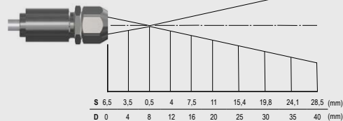
25:1 Optik mit CF-Vorsatzlinse
