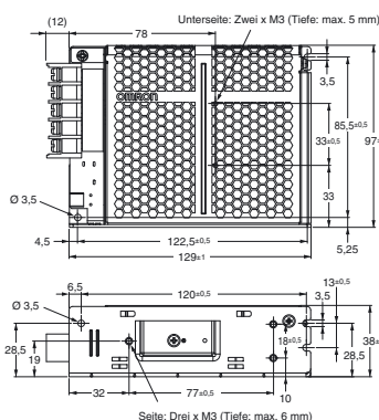
Abmessungen der Befestigungsbohrungen
