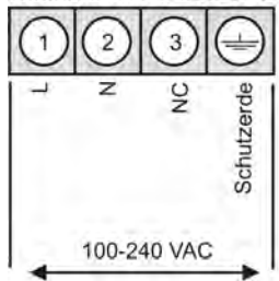
Stecker A Netzanschluss 230 VAC
