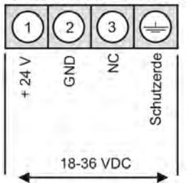
Stecker A Netzanschluss + 24 VDC
