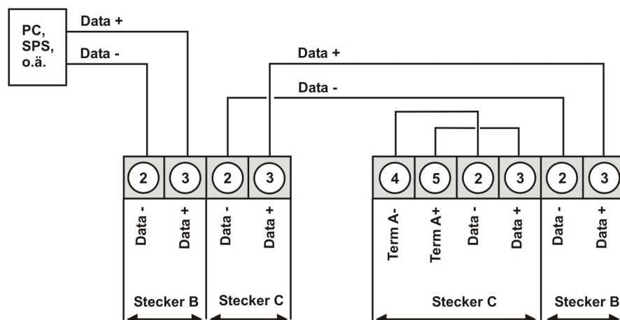
Anschluss von mehreren Anzeigen an einem Profibus - Busstrang bei MG-AB Geräten
