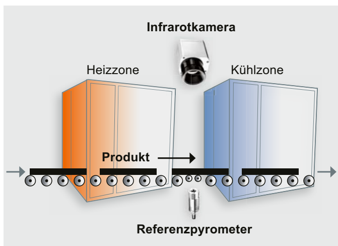
Wärmemessung an einer Glashärtungsanlage mit Infrarotkamera und Referenzpyrometer
