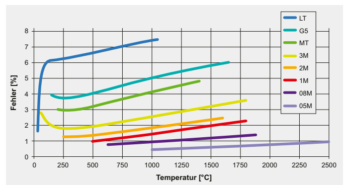
Messfehler bei 10 Prozent falsch eingestelltem Emissionsgrad in Abhängigkeit von der Wellenlänge und Objekttemperatur (LT: 8–14 μm; G5: 5 μm; MT: 3,9 μm; 3M: 2,3 μm; 2M: 1,6 μm; 1M: 1,0 μm); 08M: 800 nm; 05M: 525 nm.
