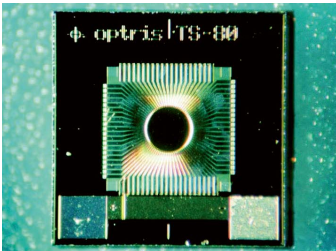
Thermosäule TS80
