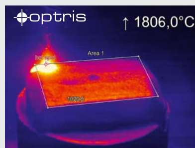
Laserschweißen
