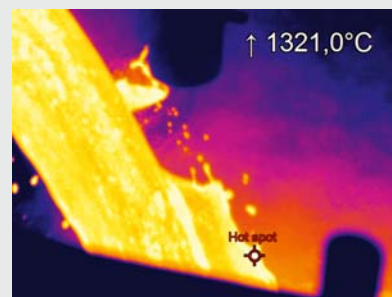
Gießstrahlmessung
