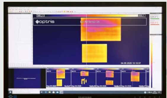
Überwachung der Temperaturen von Glasscheiben
