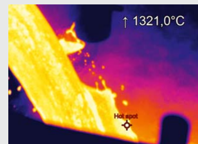
Gießstrahlmessung
