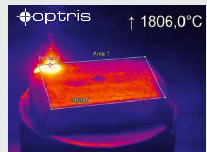
Laserschweißen
