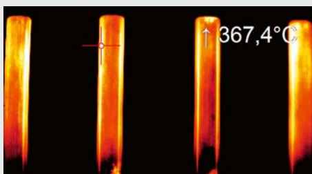
Glasröhrenherstellung
