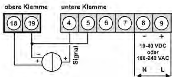
3-Leiter-Sensor 0-20 mA
