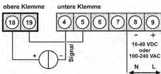
2-Leiter-Sensor 4-20 mA
