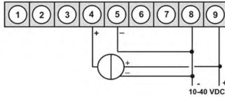
MB2-2V-Geräte in Verbindung mit einem 3-Leiter-Sensor 0/4-20 mA
